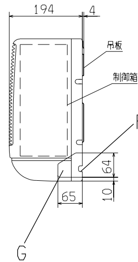
吊板詳細
