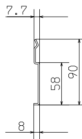
吊板詳細
