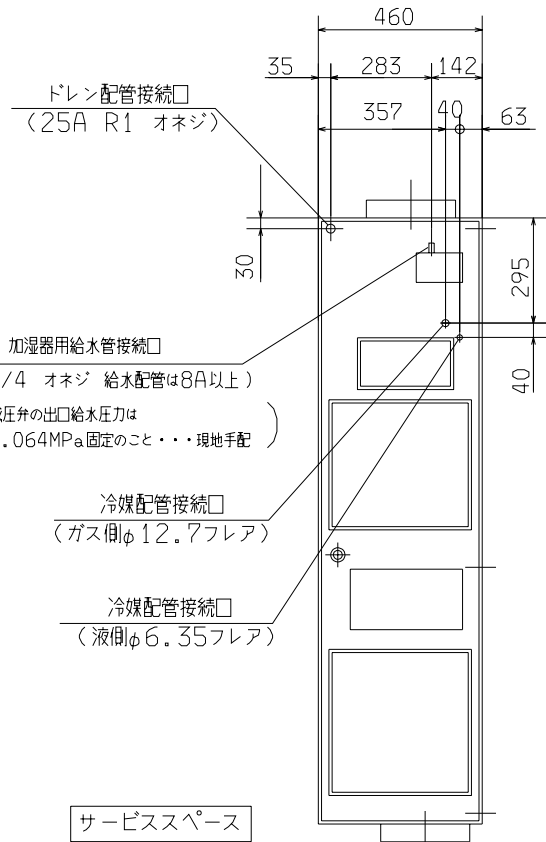
(ユニット上面より見た配置図)
