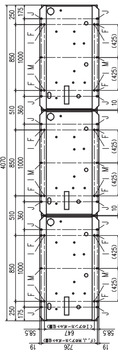
アンカーボルト用穴寸法
