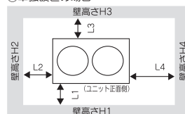
①単独設置の場合
