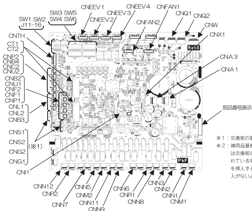
図1 部品配置図
