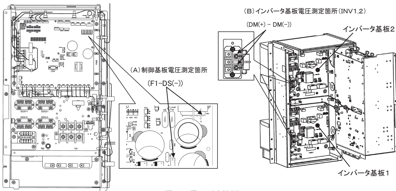
図2 電圧測定箇所
