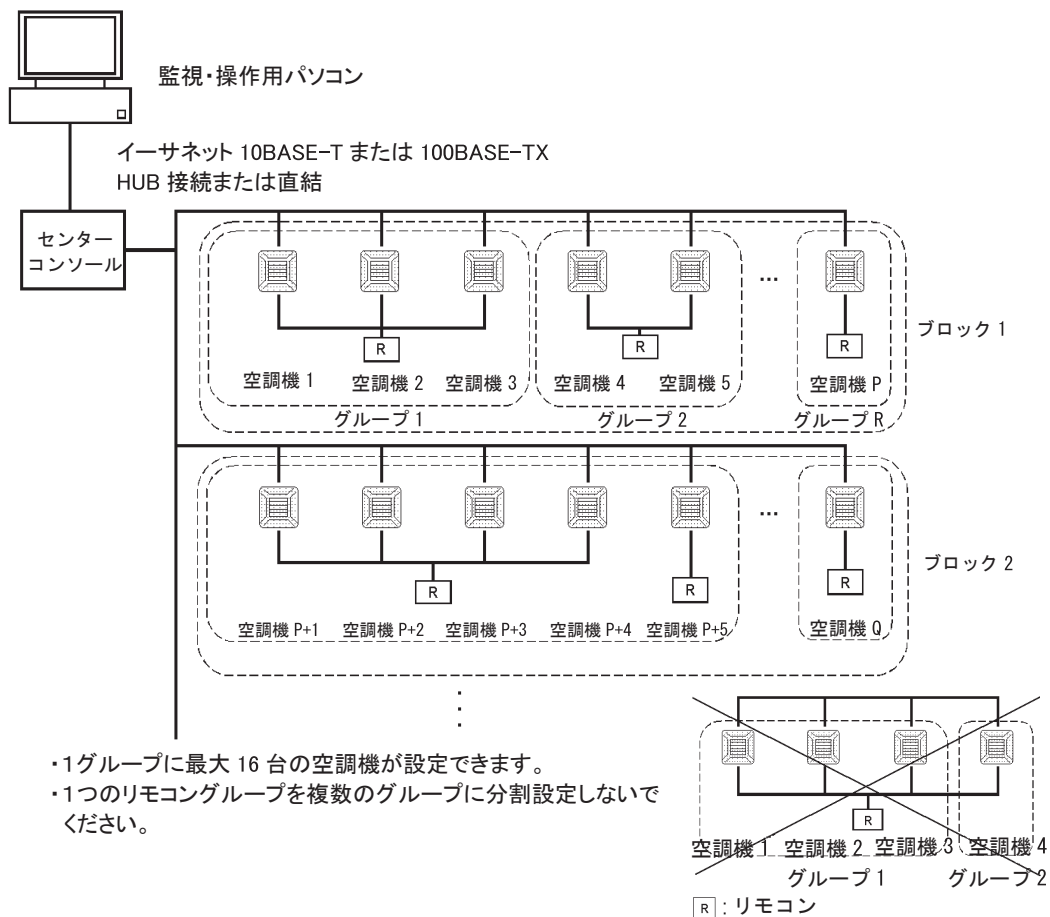
WEB 監視システム構成図
