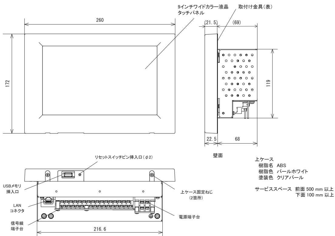
(a) 本体
