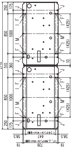
アンカーボルト用穴寸法
