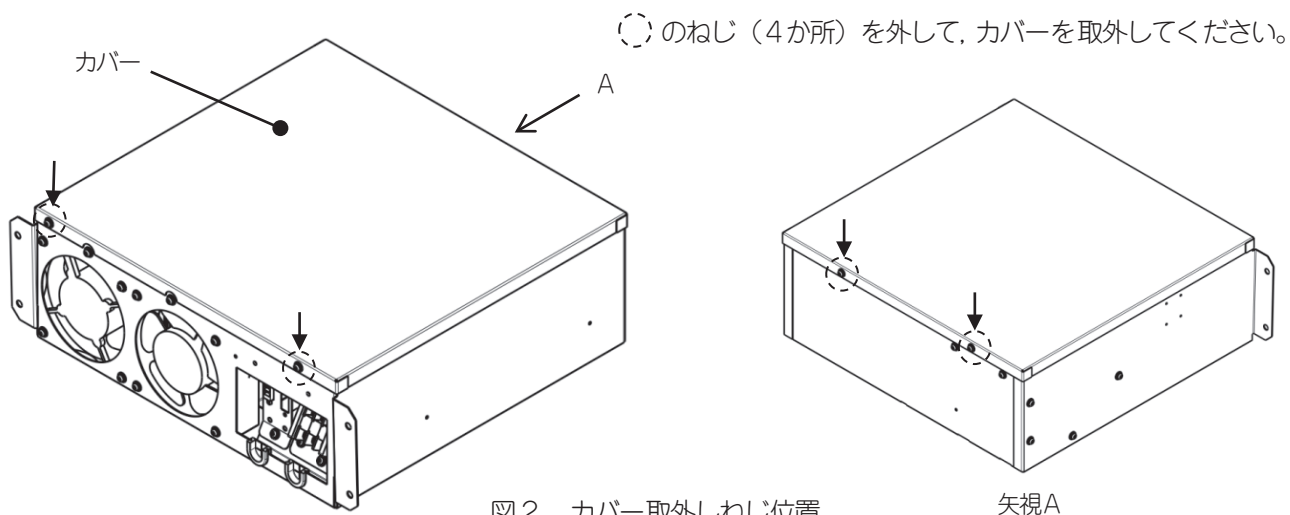
図2 カバー取外しねじ位置
