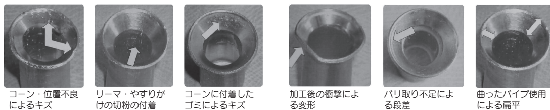
図2 フレア加工の不具合例
