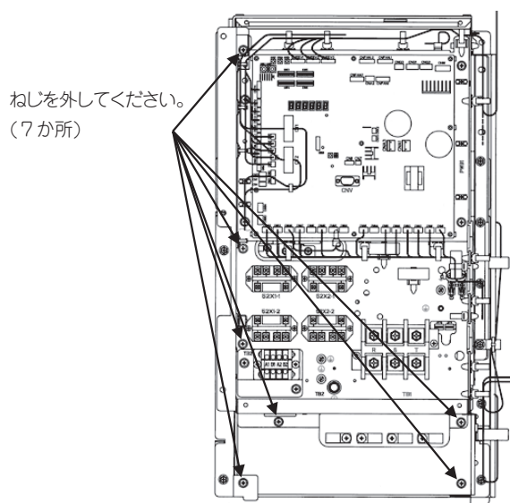
図3 取外し箇所
