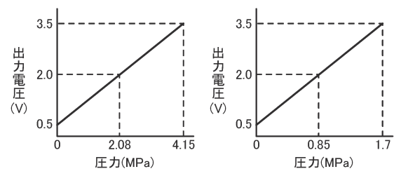
高圧圧力センサ出力特性 低圧圧力センサ出力特性
