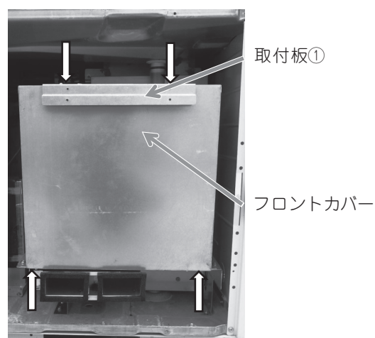
図3 AF搭載状態（カバー②取外し後）
